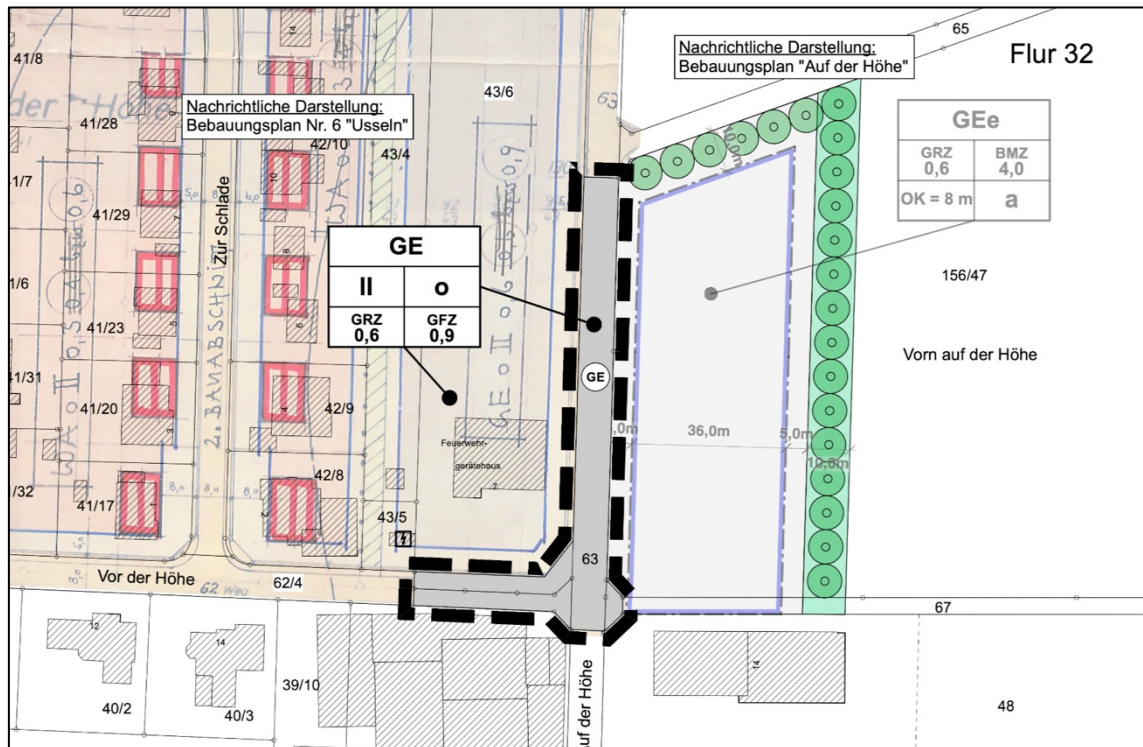
Abbildung 8: B-Plan „Usseln, 2. Änderung“ - Planteil
