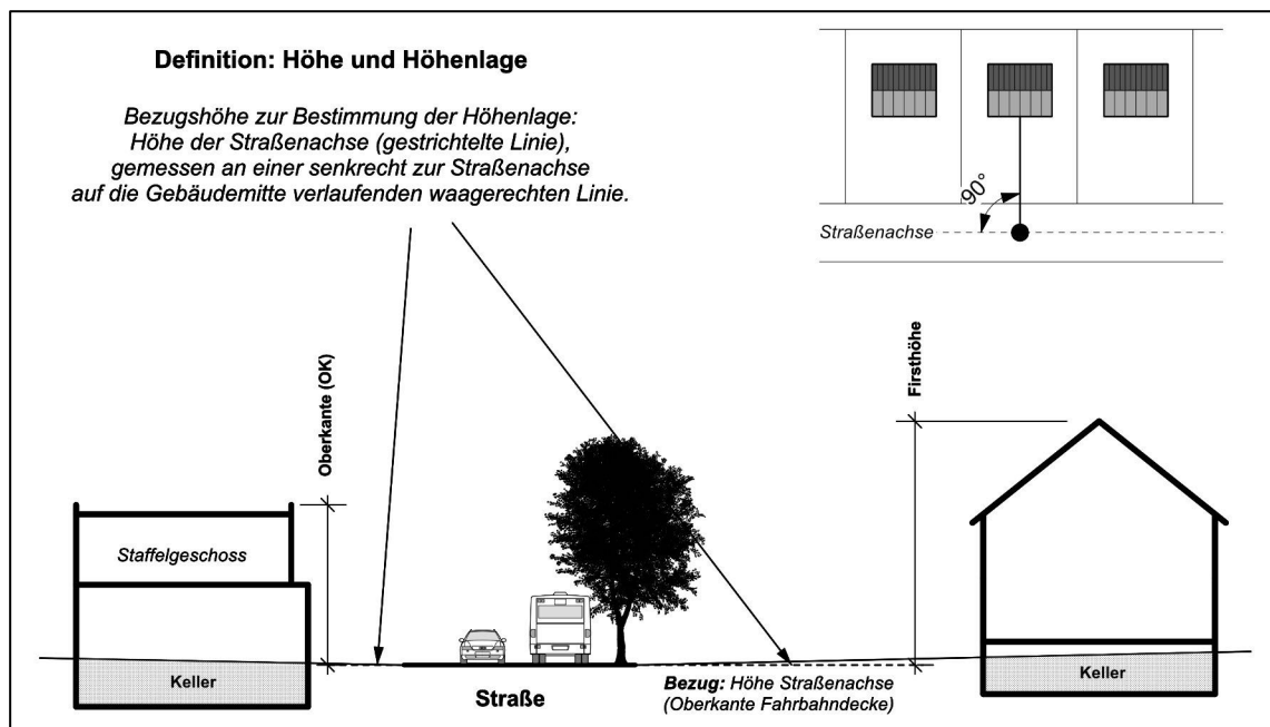
Abbildung 13: Definition zur Höhe und Höhenlage - eigene Skizze
