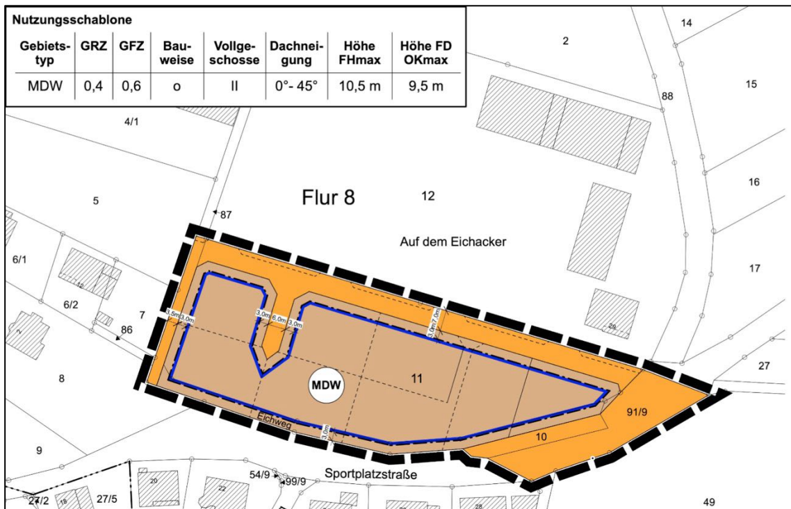
Abbildung 12: Bebauungsplan – Planteil
